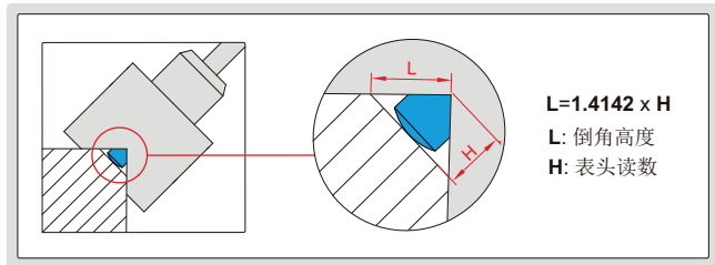
测量原理
